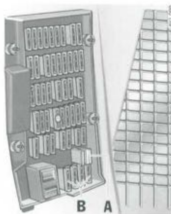
A - Pince isolante B - Fusibles de remplacement
