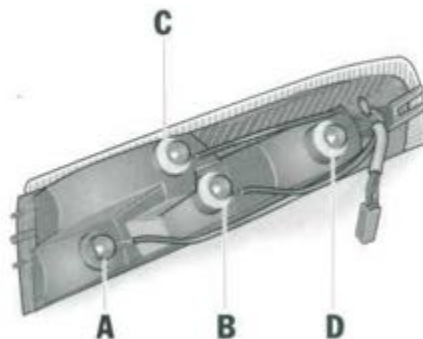
A - Feu arrière / feu stop B - Feu de recul C - Clignotant D - Feu arrière de brouillard
