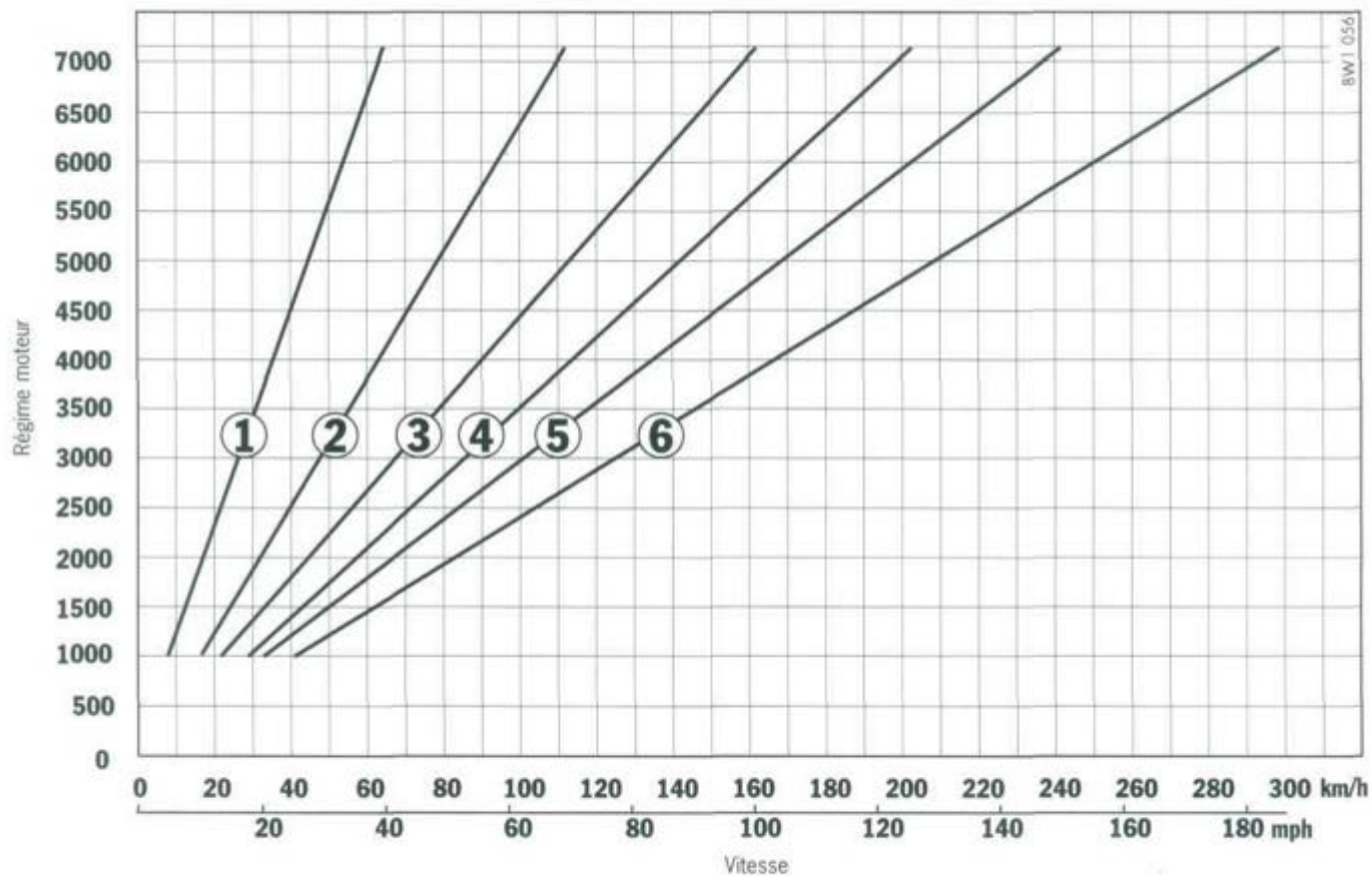
Diagramme de transmission Boîte mécanique
