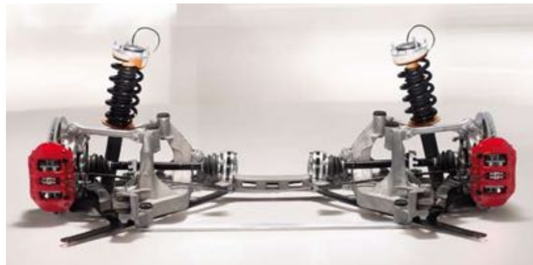
Essieu arrière de la 911 Turbo
