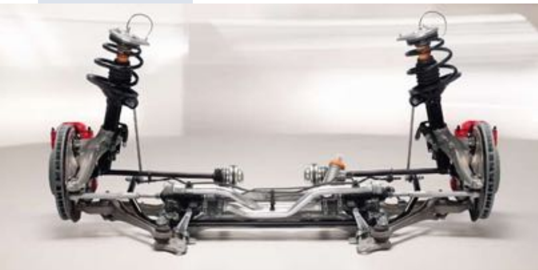
Essieu avant de la 911 Turbo
