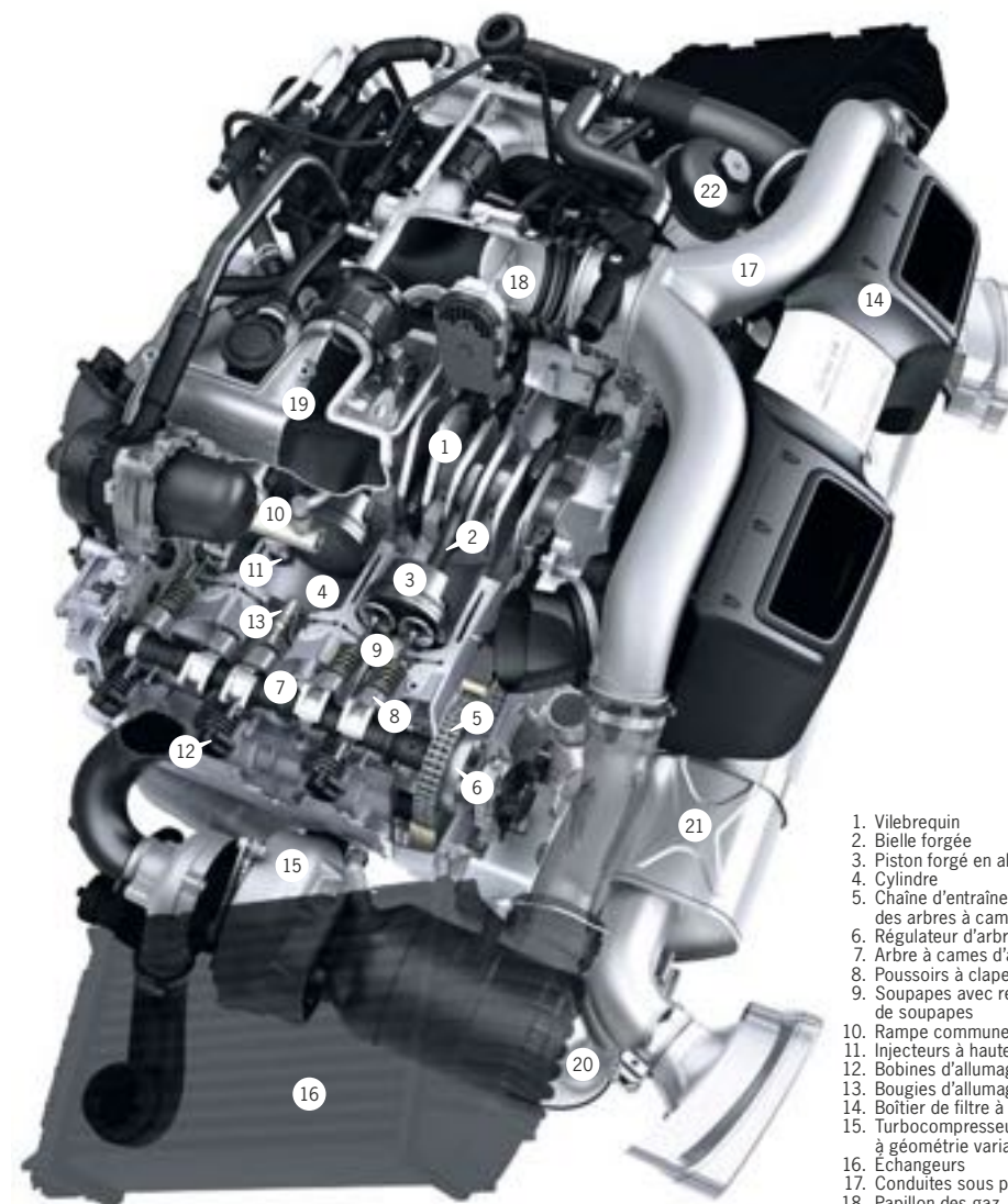
Moteur avec boîtier de filtre à air en carbone des nouveaux modèles 911 Turbo S
