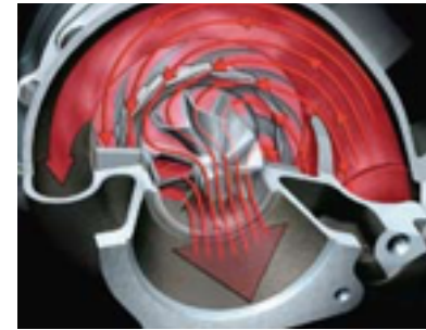
Ailettes orientables fermées
