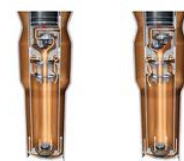
Phase de compression – Piston plus by-pass = réglage sportif confortable
